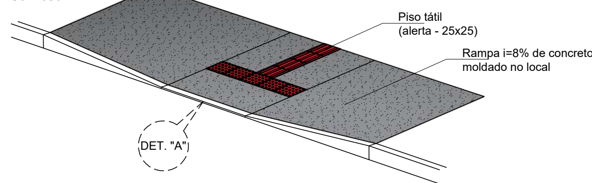
PERSPECTIVA Sem esc.
