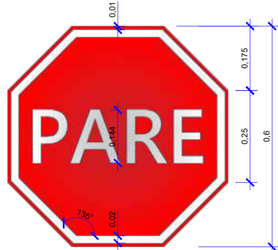
DETALHE DE PLACA - R1 ESC. 1:10
