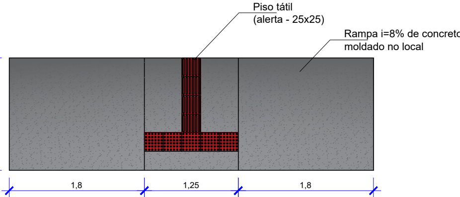
DETALHE "A" Sem esc.
