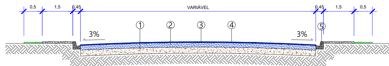
SECÇÃO TRANSVERSAL SEM ESCALA
