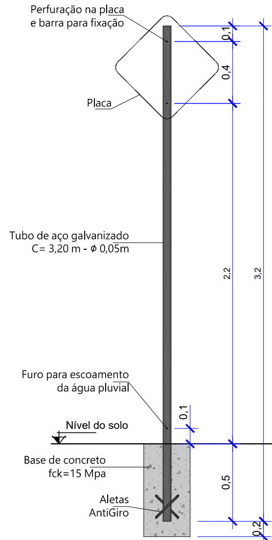
VISTA - POSTE ESC. 1:25
