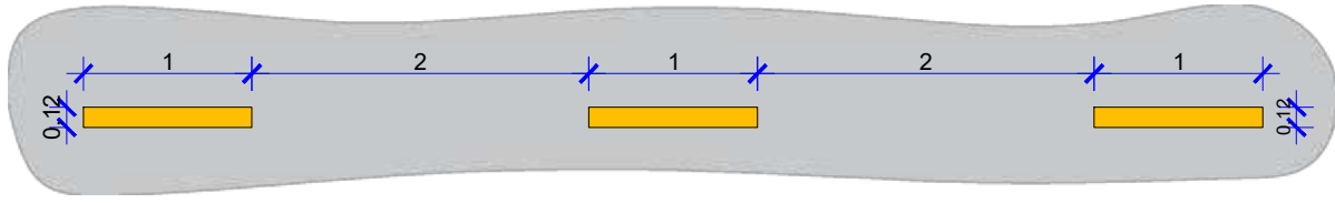
DETALHE GENÉRICO - FAIXA SEGMENTADA AMARELA ESP. = 12 CM - AFAST. = 1,00 M x 2,00 M ESC.1:50
