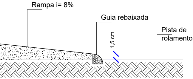
DETALHE "A" Sem esc.
