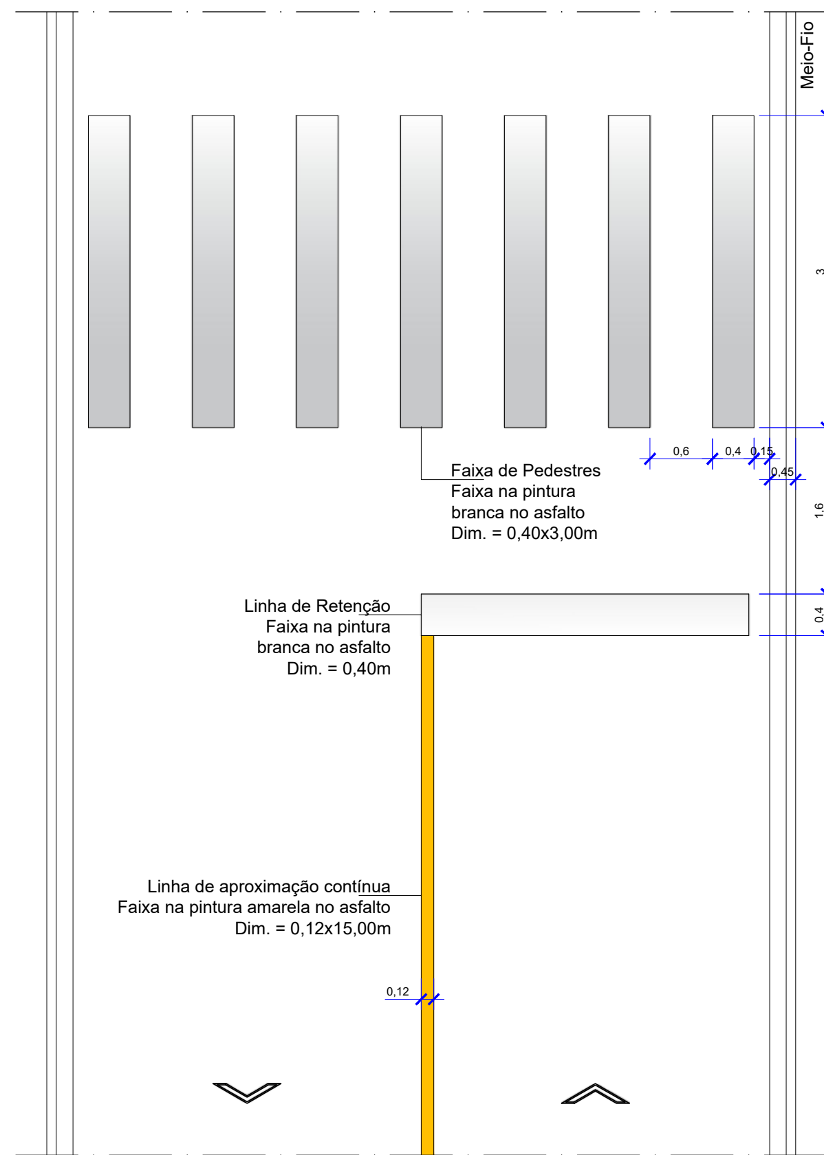
DETALHE GENÉRICO - SINALIZAÇÃO HORIZONTAL ESC. 1:50
