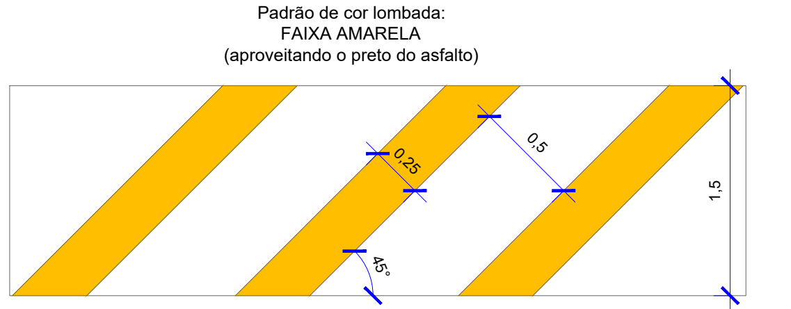
DETALHE - SINALIZAÇÃO HORIZONTAL ( LOMBADA ) ESC.1:25
