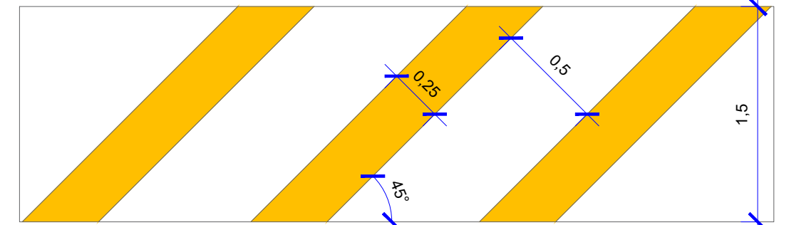
DETALHE - SINALIZAÇÃO HORIZONTAL ( LOMBADA ) ESC. 1:25
