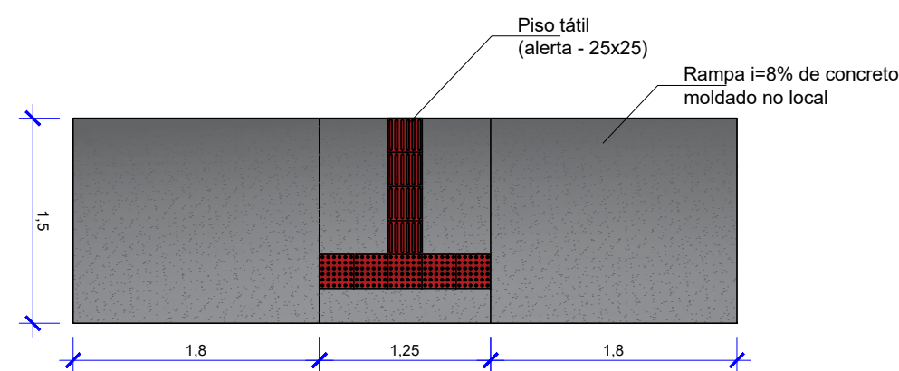
PLANTA BAIXA - RAMPa P.N.E. ESC. 1:50
