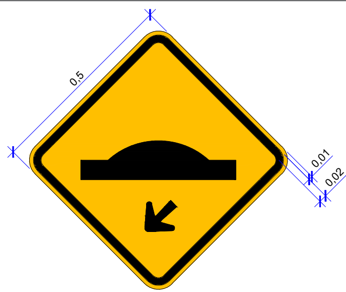
DETALHE - PLACA A-18 ( Saliência ou lombada ) ESC. 1:10
